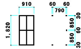
吊り棚 詳細図 S=1/50
