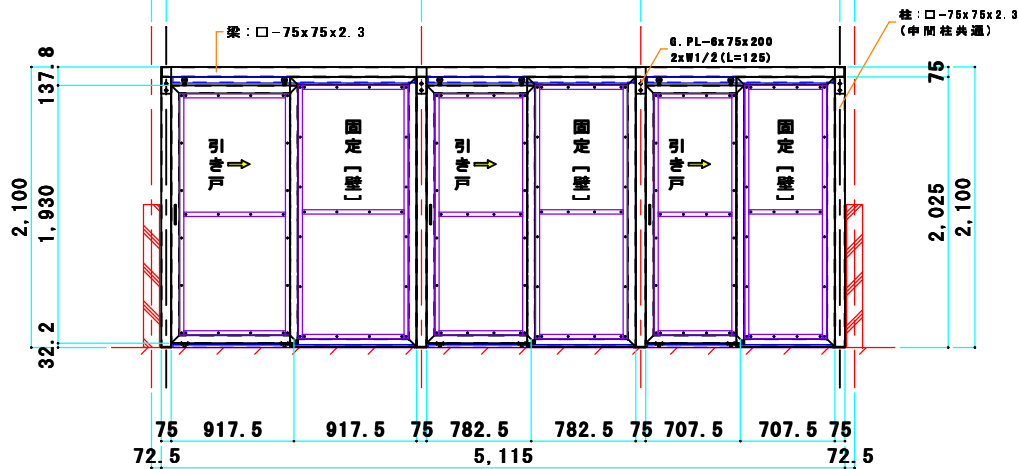
立面図 S=1/20
