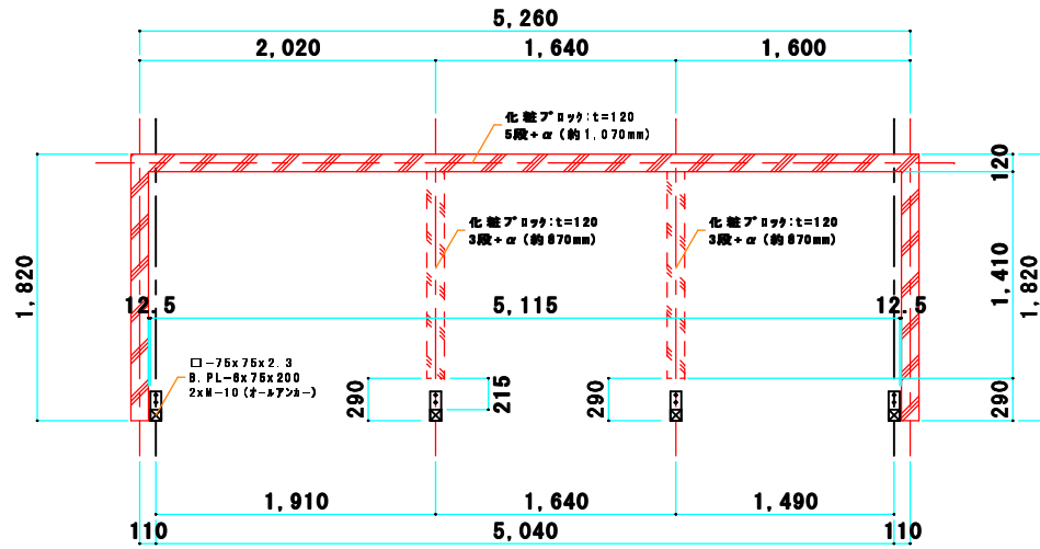
平面図 S=1/20
